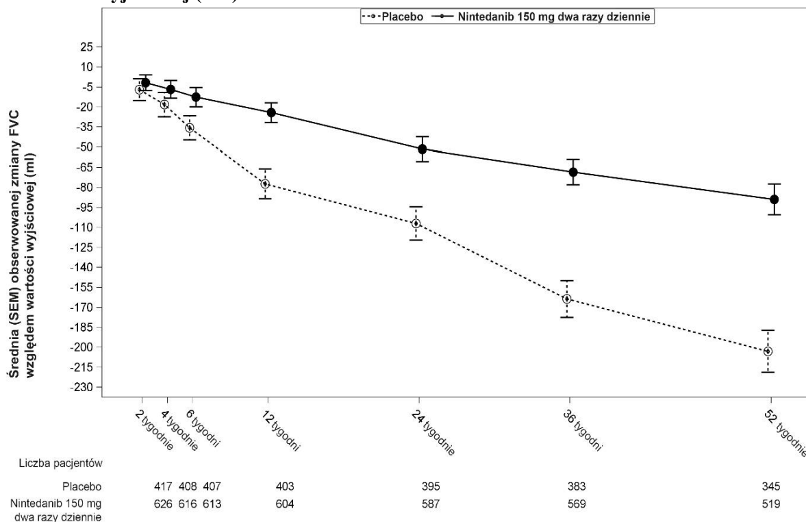
Rycina 1: Średnia (SEM) zaobserwowana zmiana FVC z stosunku do wartości wyjściowej (mL) w czasie - zbiorcze dane z badań INPULSIS-1 i INPULSIS-2
